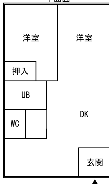
平面図
