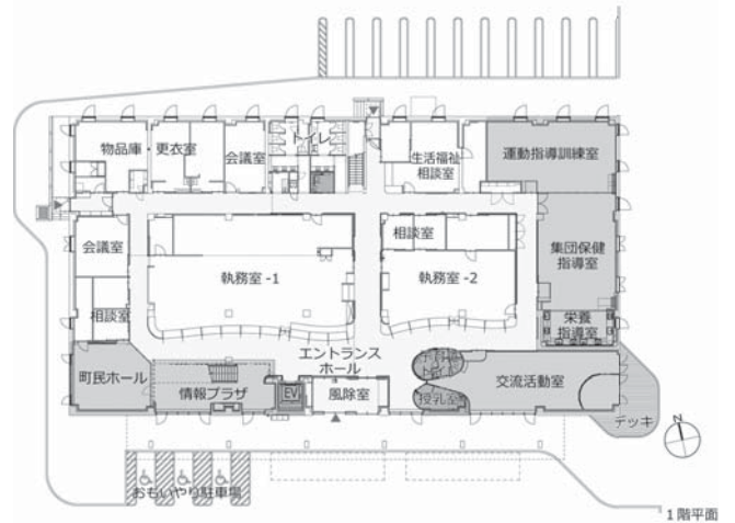
1階平面
