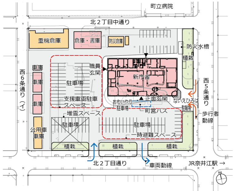
配置計画
