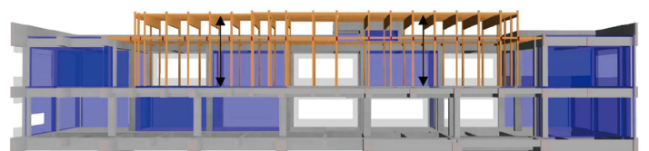
構造架構断面パース（全体）
