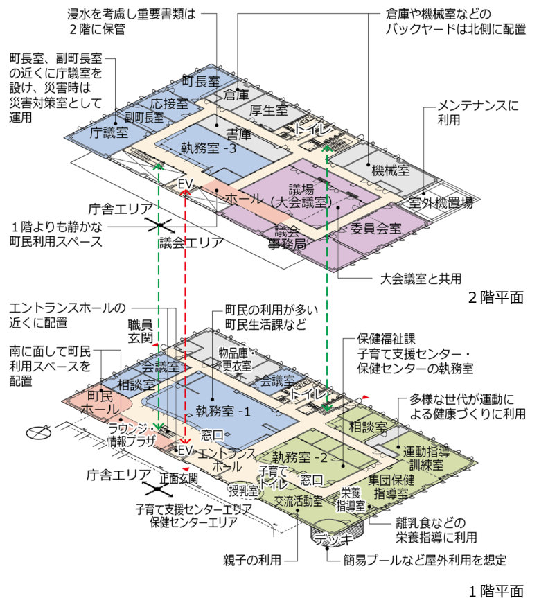
1階平面
